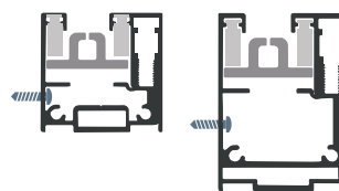
EXTERNE INSTALLATIE OP DE VOORKANT, MET RAILS DIE FRONTAAL BEVESTIGD ZIJN
