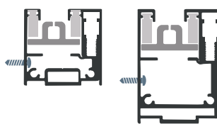
INSTALLAZIONE ESTERNA FRONTALE CON FISSAGGIO FRONTALE DELLE GUIDE
