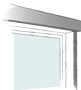
INSTALLAZIONE ESTERNA FRONTALE CON FISSAGGIO FRONTALE DELLE GUIDE
